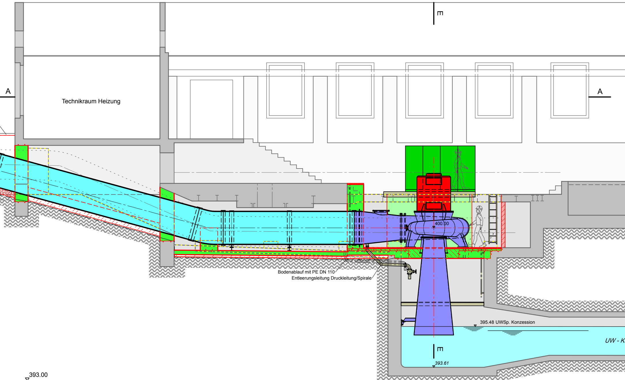
Kraftwerk WebCenter Aarburg Längsschnitt D - D
