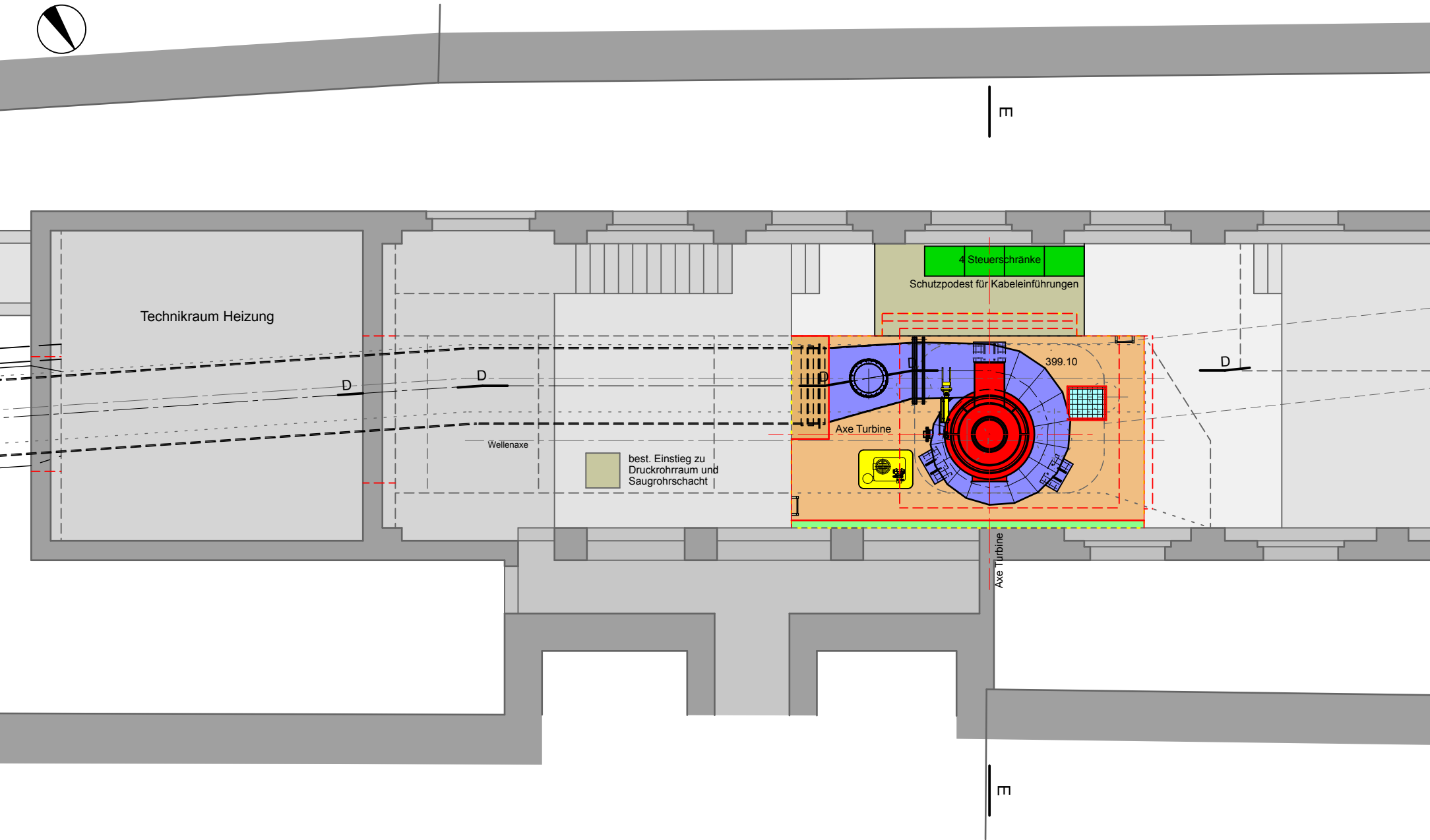
Kraftwerk WebCenter Aarburg Horizontalschnitt A - A
